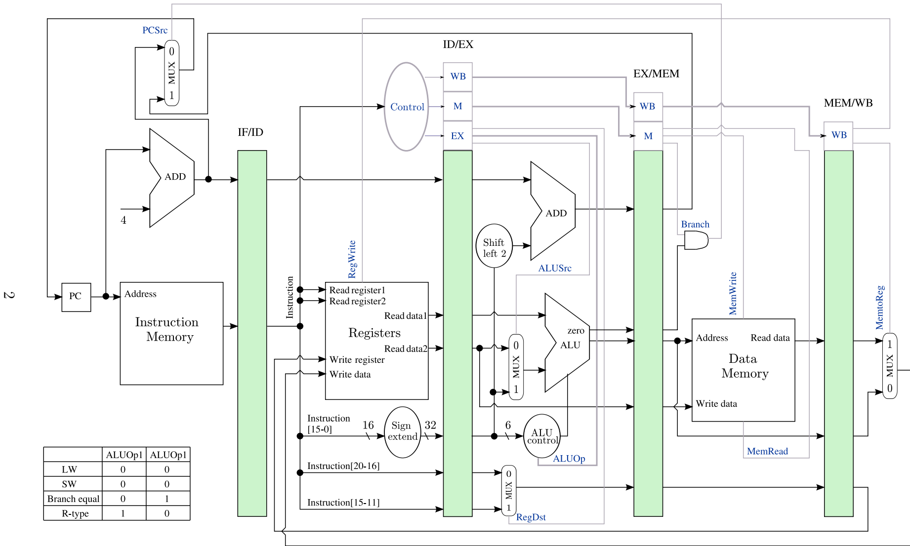
Abbildung 1: Datenfad, Kontrolleinheiten und Steuersignale der Pipeline-CPU.
