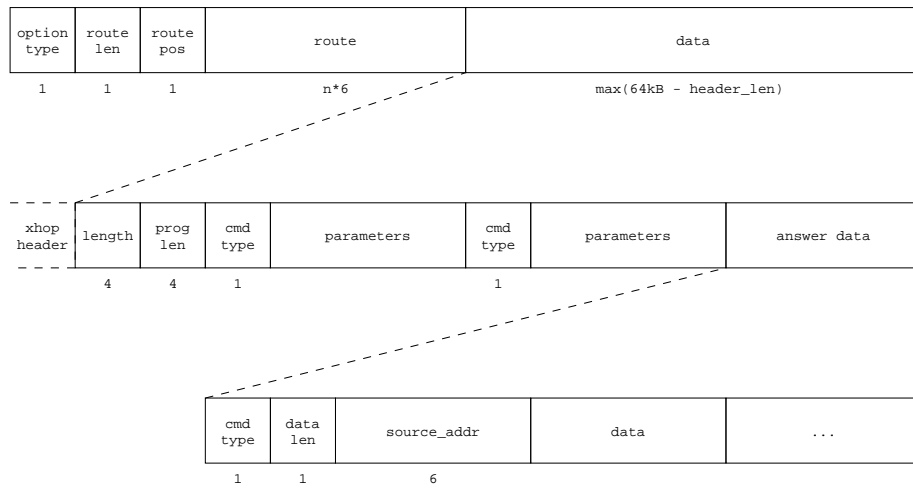
Abbildung 3.1: Paketformat von xhop
